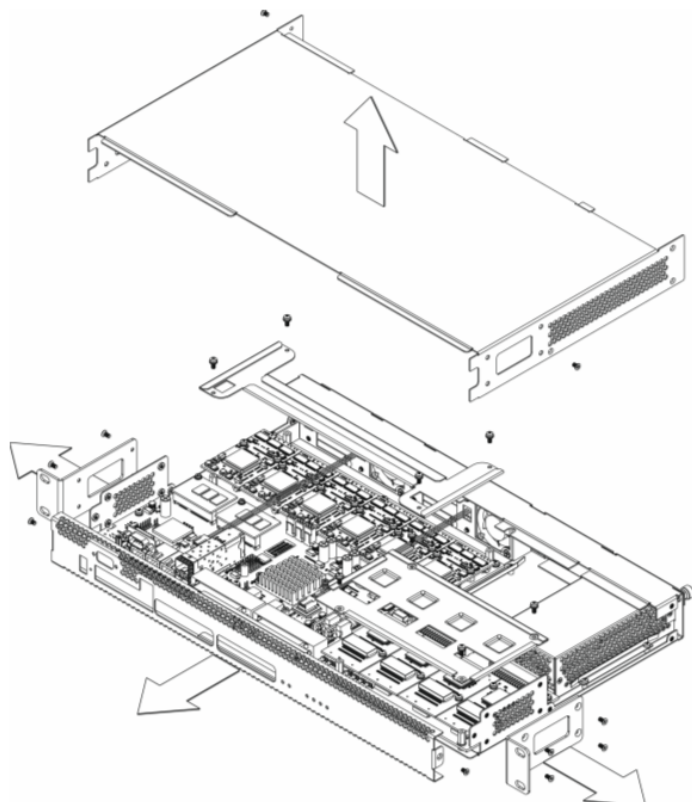
Рисунок 22 – Порядок вскрытия корпуса SMG-1016M
