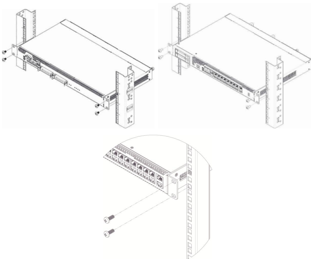
Рисунок 20 – Установка устройства в стойку SMG-1016M (слева), SMG-2016 (справа) и SMG-3016 (внизу)
