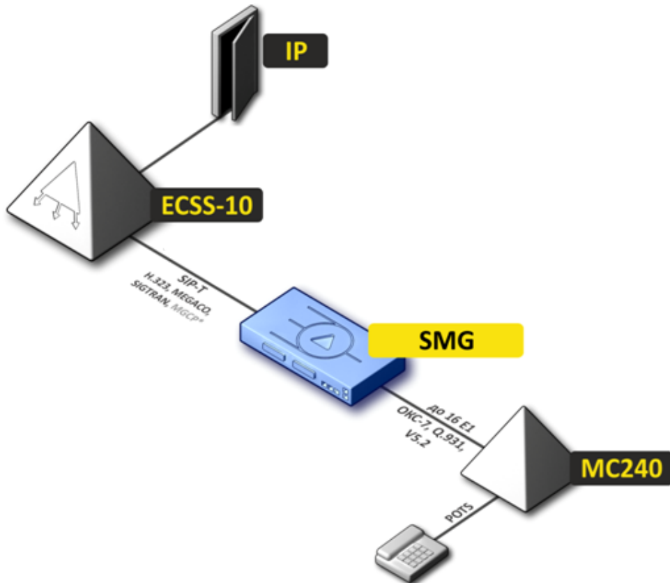
Рисунок 2 – Сопряжение сигнализаций и медиа-поточков TDM и VoIP сетей
