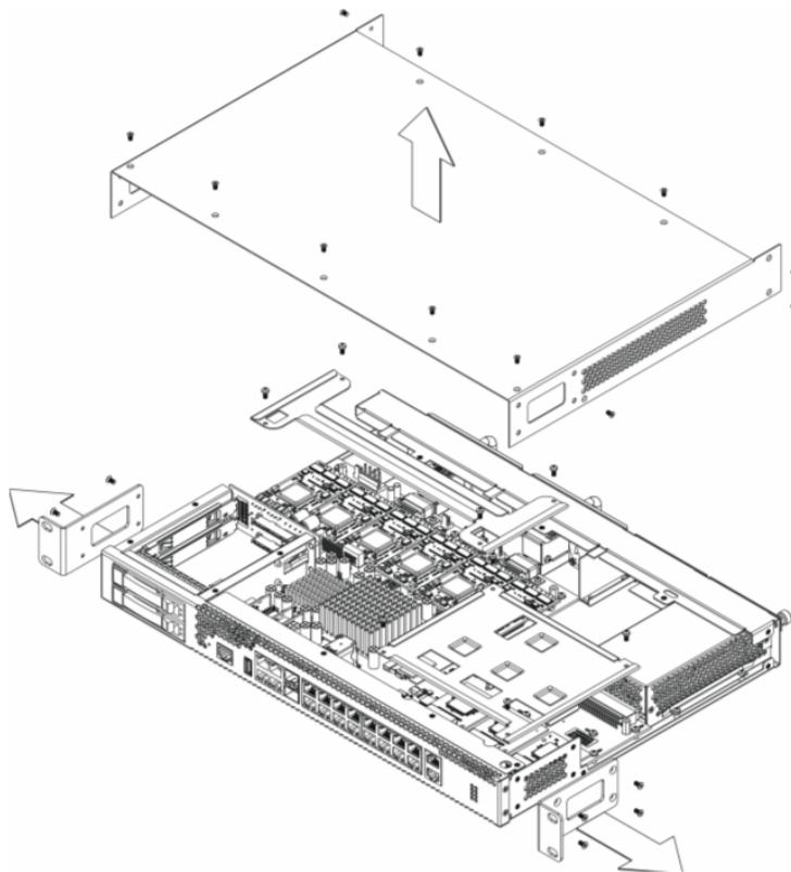
Рисунок 23 – Порядок вскрытия корпуса SMG-2016
