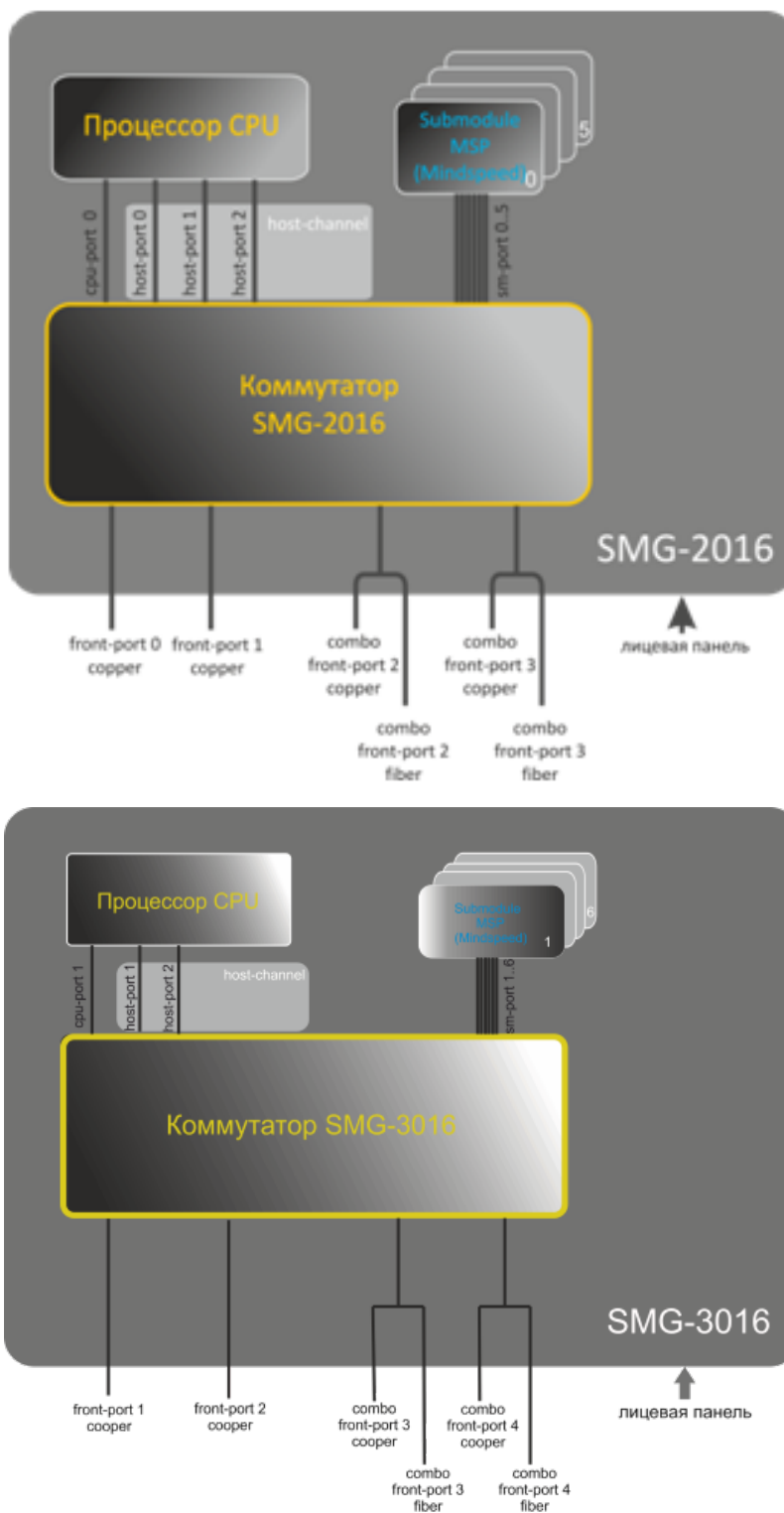
Рисунок 49 – Структура коммутатора
