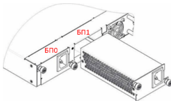
Рисунок 21 – Установка модулей питания
