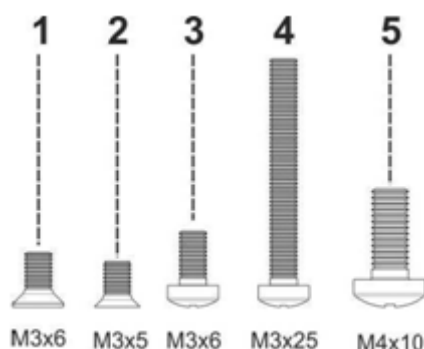
Рисунок 25 – Типы болтов для сборки SMG
