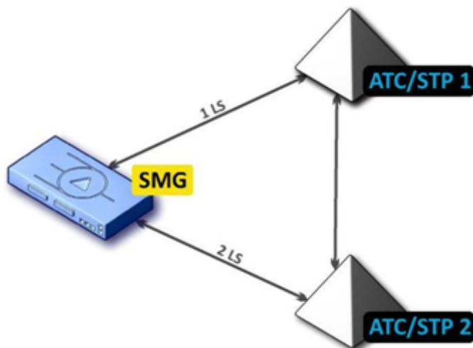
Рисунок 47 – Схема подключения SMG при работе в квазисвязанном режиме через АТС с STP
